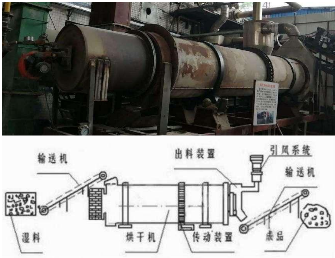
图 3.3-5 天然气烘干炉示意图
