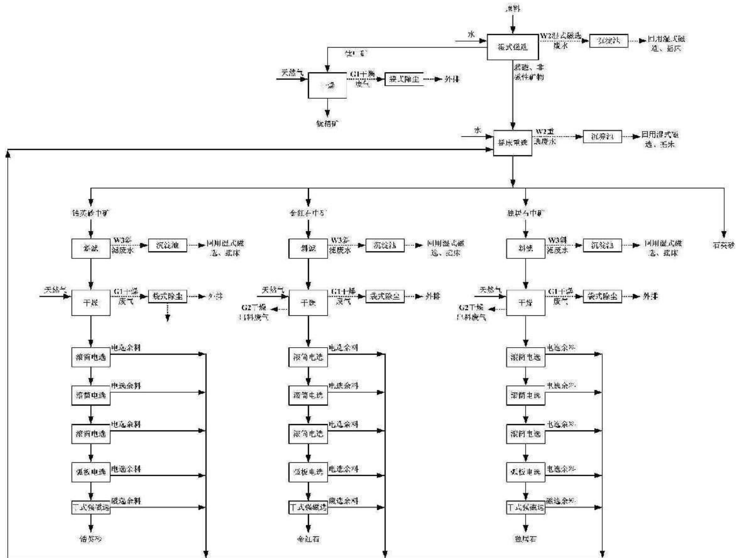
图 3.3-6 项目生产工艺流程及产污环节图
