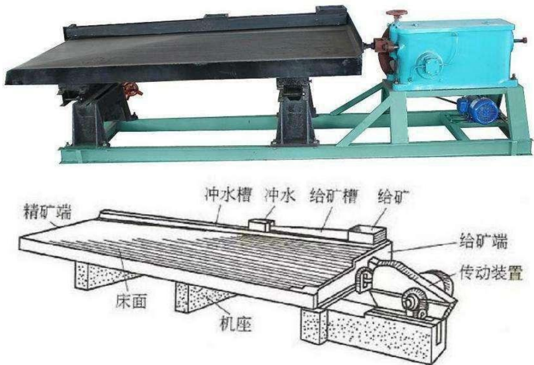
图 3.3-3 摇床结构示意图
