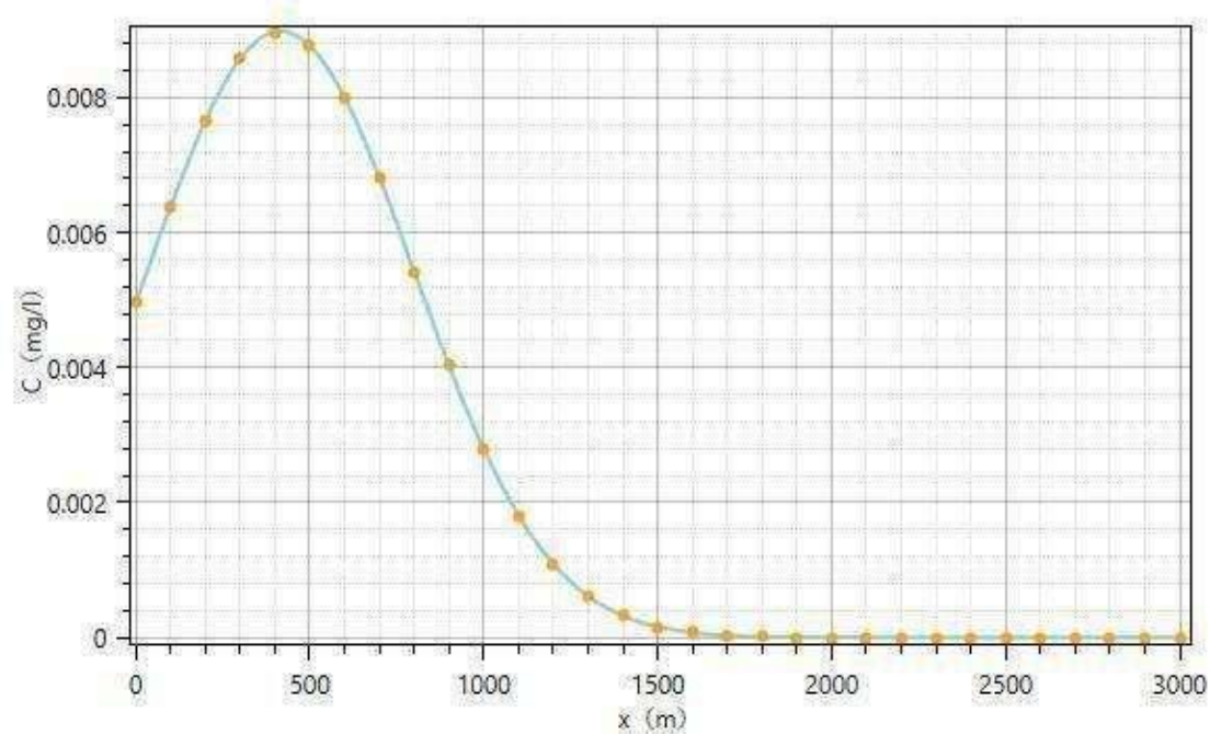
图 5.6-8 时间 T=7300d ，泄漏氨氮迁移预测结果图
