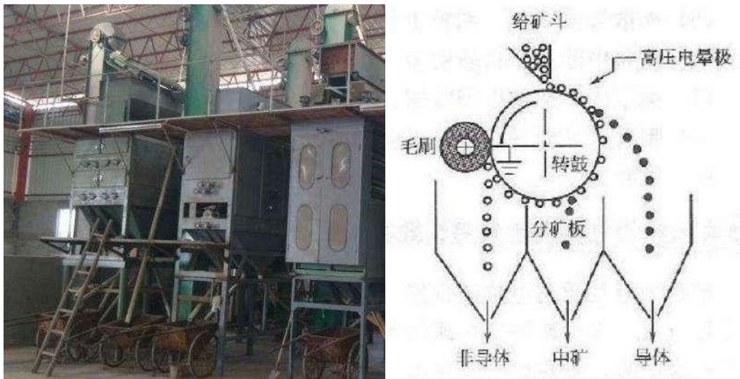
图 3.3-4 电选机结构示意图
