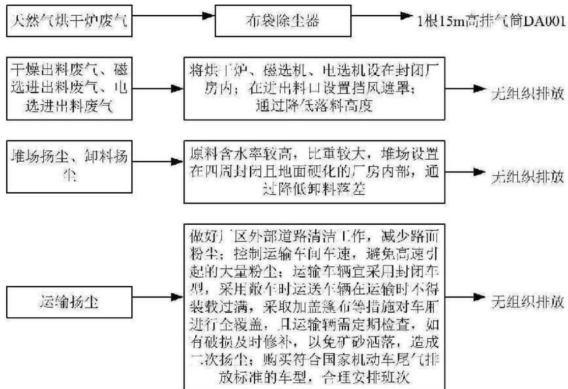
图 6.2-1 项目废气处理工艺流程图
