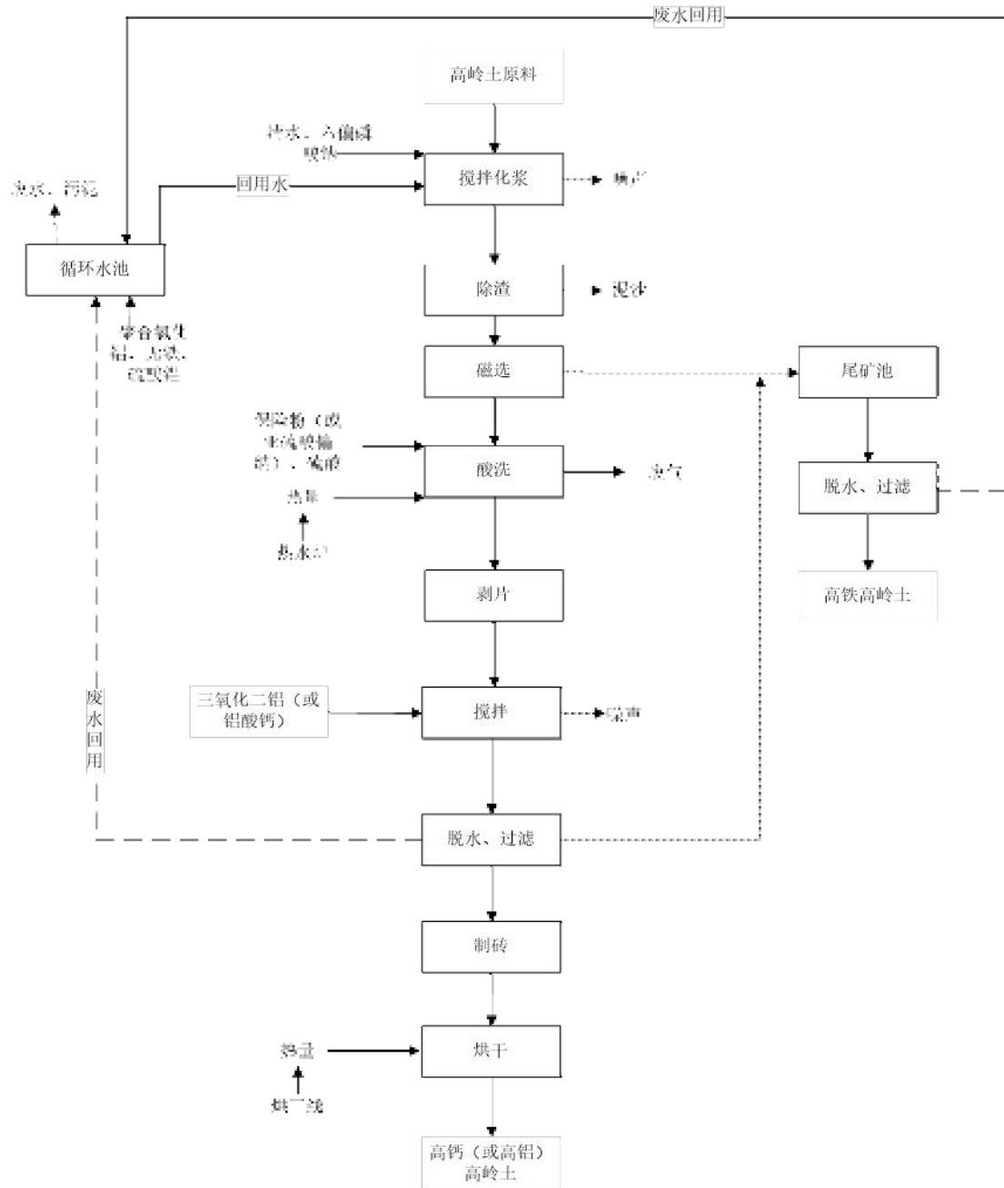
图 3.1-3 原环评高钙、高铝高岭土生产工艺流程图
