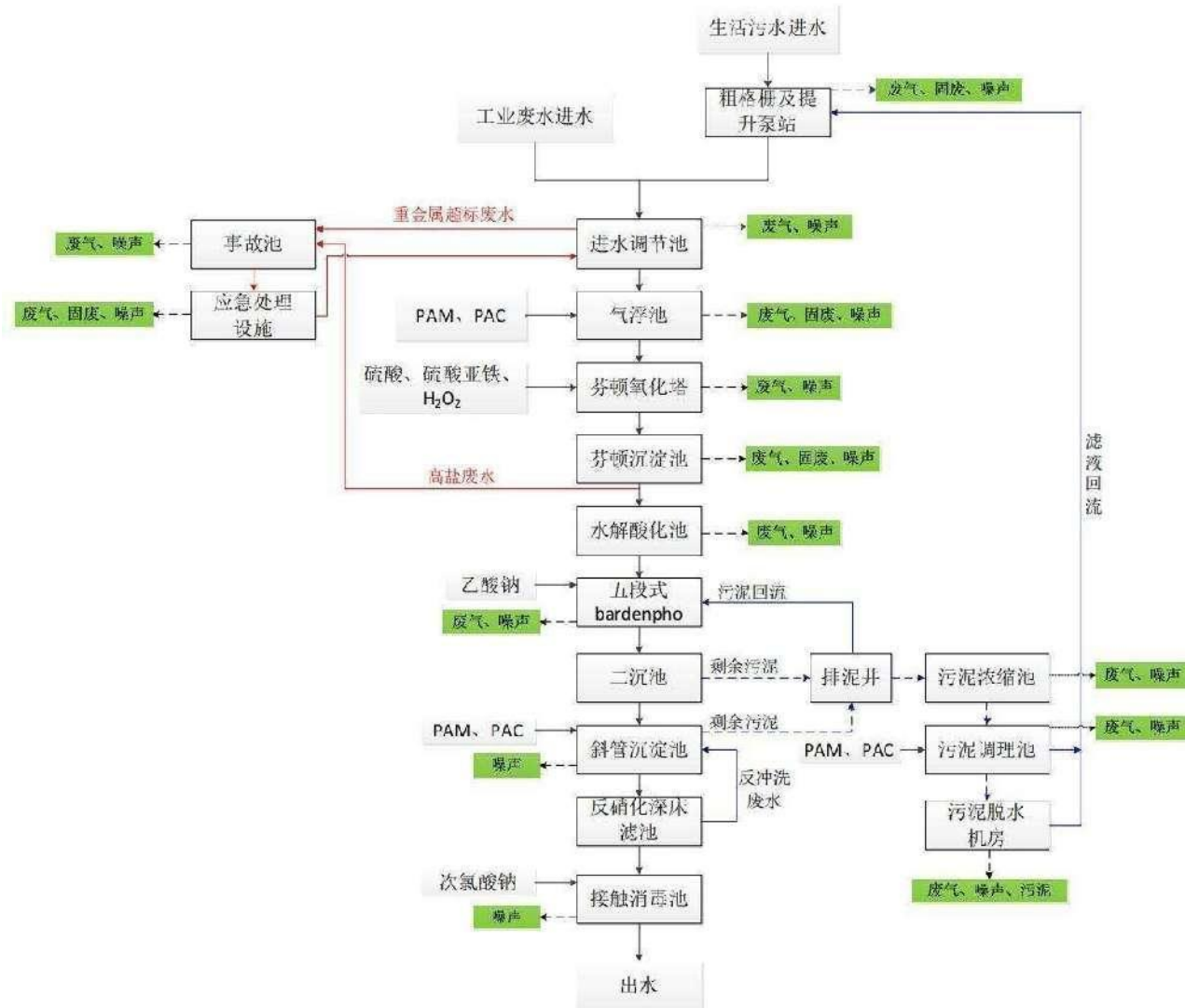
图 6.1-2 漳浦县赤湖工业园五金园区污水处理厂污水处理工艺流程图
