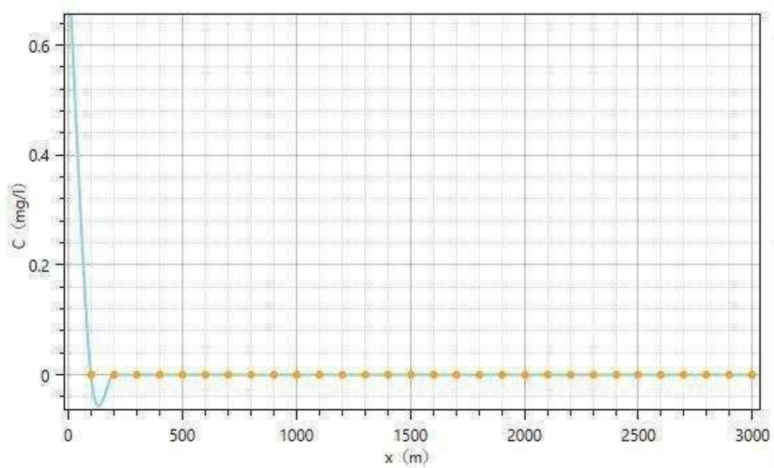
图 5.6-5 时间 T=1d ，泄漏氨氮迁移预测结果图
