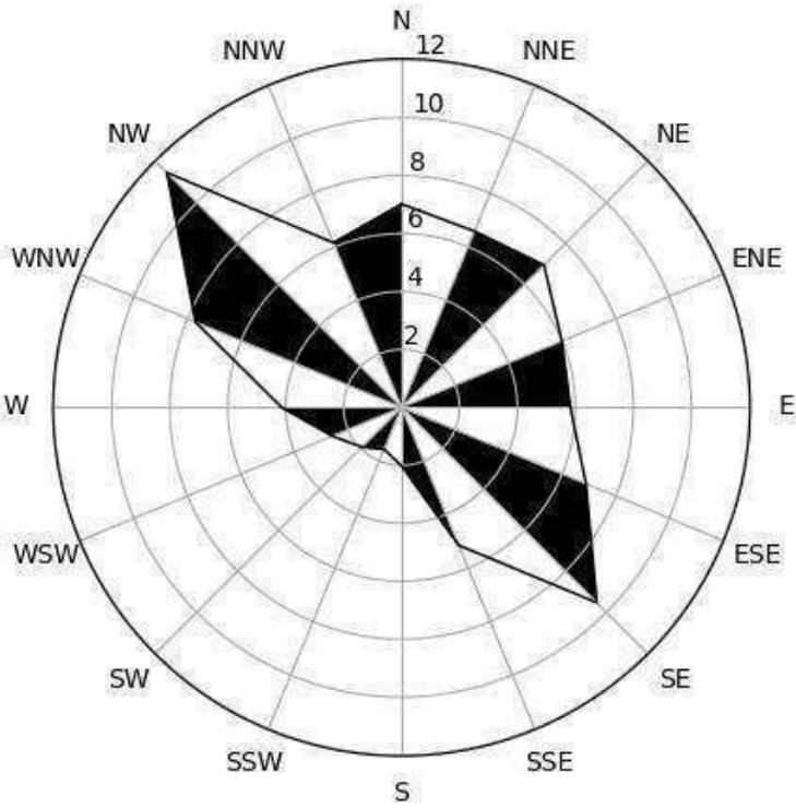
图 5.2-1 漳浦风向玫瑰图（静风频率 7.79%）
