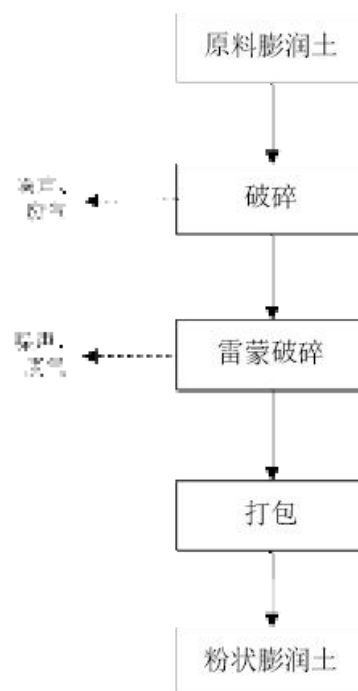
图 3.1-2 原环评粉状膨润土生产工艺流程图
