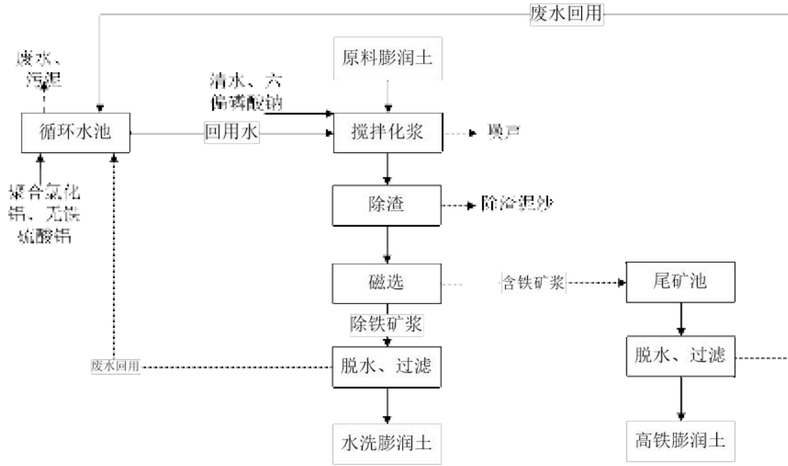
图 3.1-1 原环评水洗膨润土生产工艺流程图
