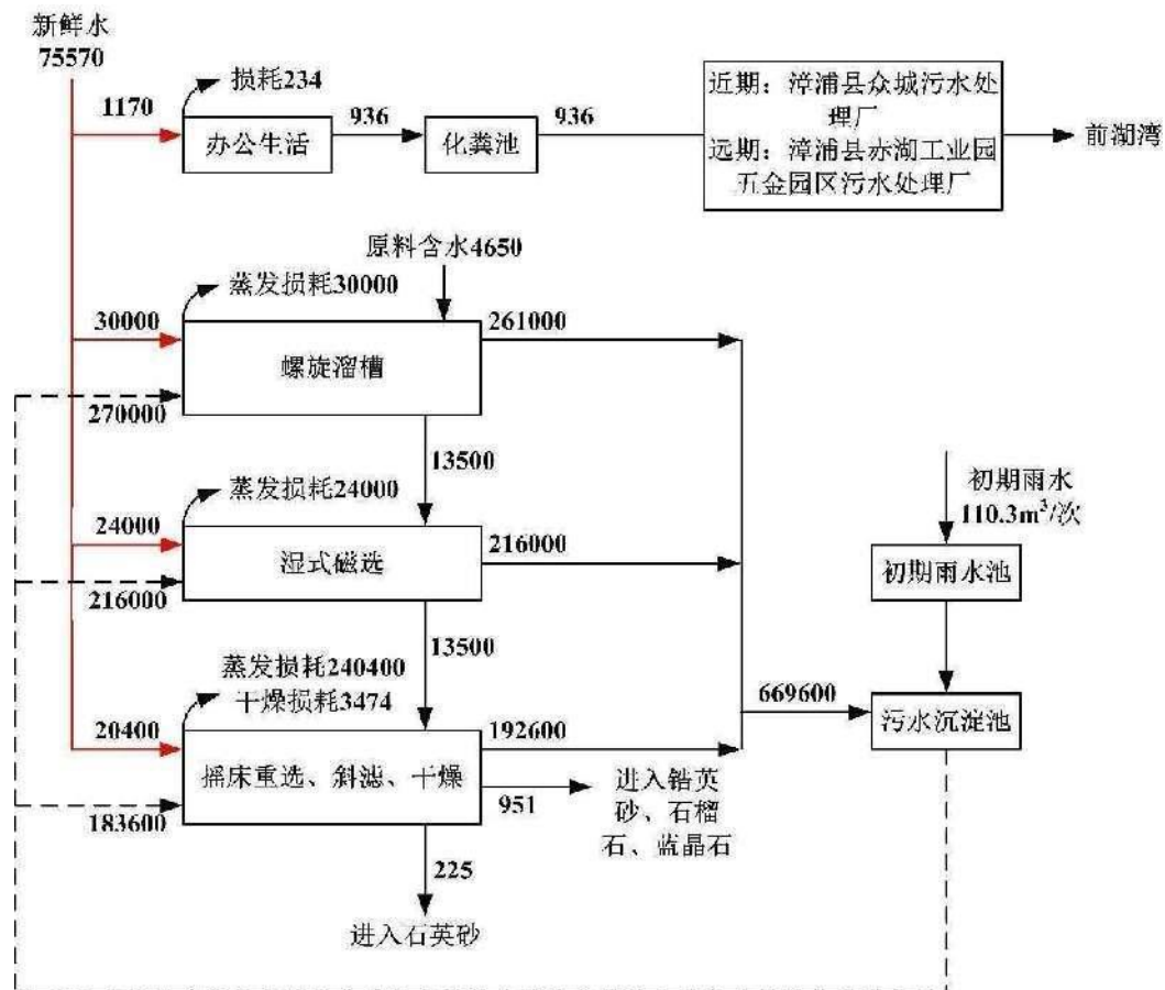
图 3.3-8 项目水平衡图 (t/a)
