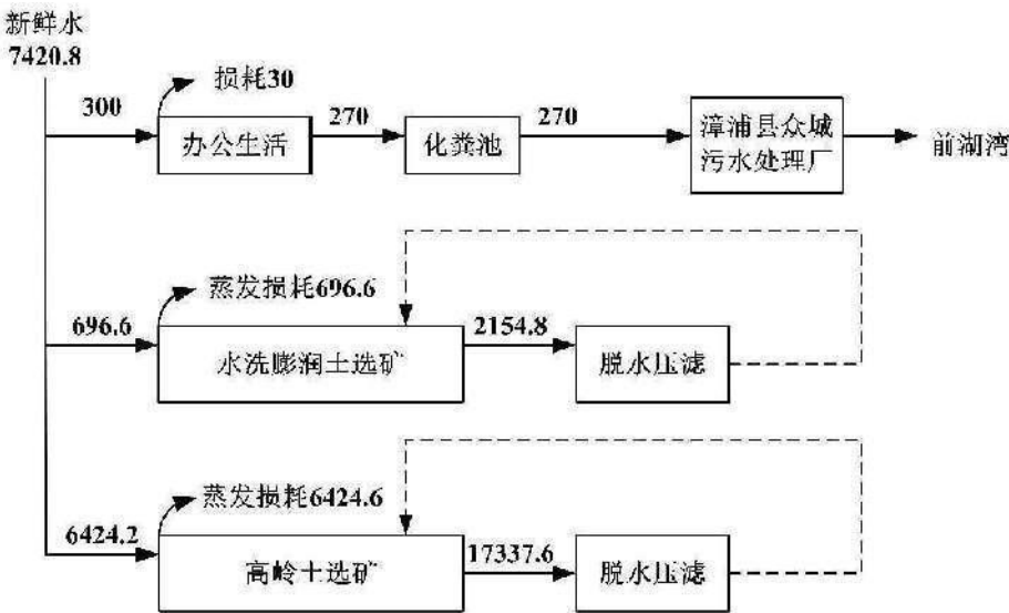
图 3.1-5 现有工程水平衡图 (t/a)
