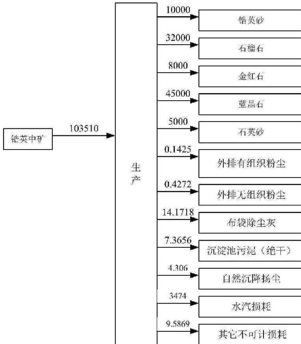
图 3.3-7 项目全厂物料平衡图 (t/a)
